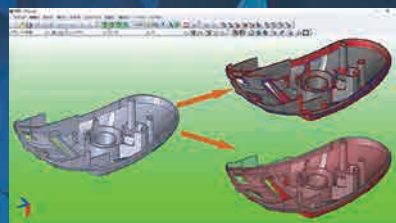
[シャドウ面・肉厚色分け機能]
