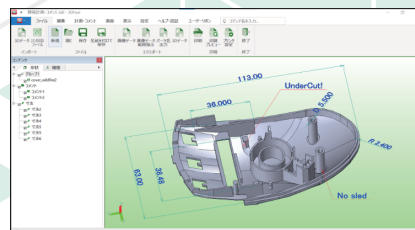
計測・コメント機能
